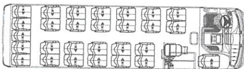
Planta do modelo Attack 8
