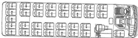
Planta do modelo Attack 9
